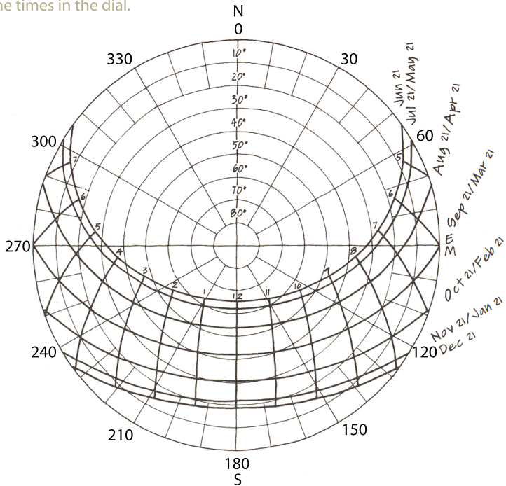
Sun Path Diagram, 48° Latitude
